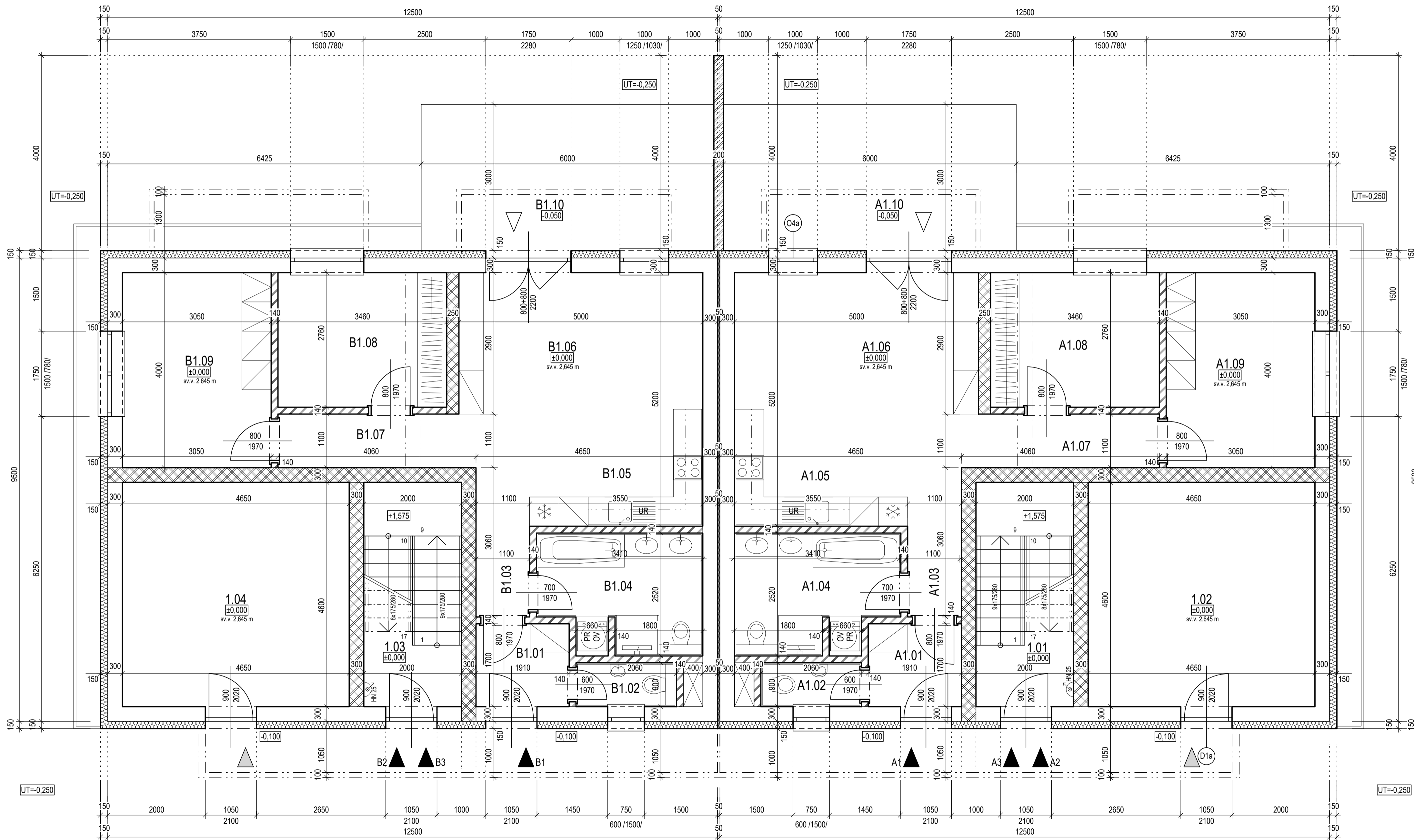
PÔDORYS 1.N.P. M1:50
